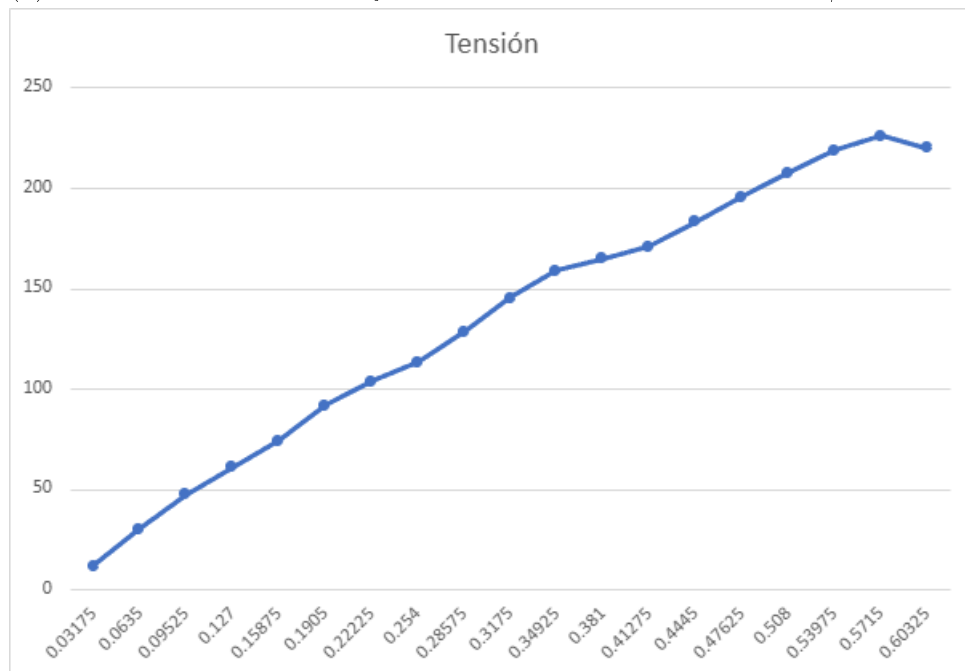
(b) Gráfica obtenida del ensayo de tracción del alambre de aluminio AA 1305 H19.
