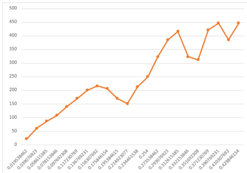
(a) Gráfica obtenida del ensayo de tracción del hilo de acero SAE/AISI 1045.
